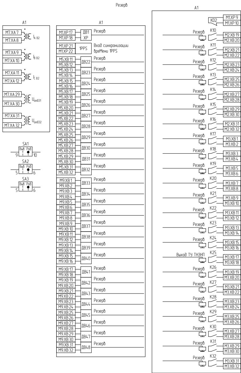
Рисунок Г.3 – Схема электрическая принципиальная (часть 3)
