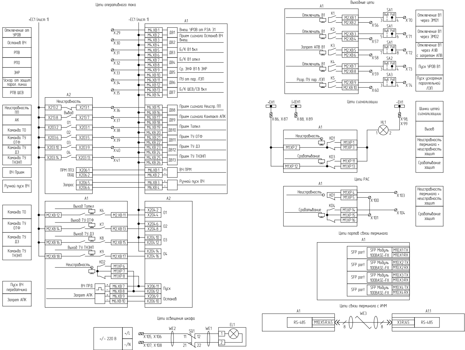
Рисунок Г.2 – Схема электрическая принципиальная (часть 2)
